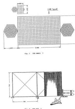
図 2 第 2 回の宇宙エネルギーシンポジウムでの長友先生のご講演 ”Introductory Note on the 10 MWSPS Conceptual Study”で示された 10MW 級 SPS の大きさ
