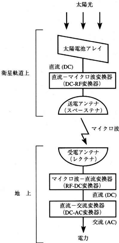
第1図 宇宙発電所と地上受電設備の基本的な構成 (1) 。 宇宙発電所では太陽エネルギーを利用して発電し、電気エネルギーをマイクロ波に変換して地上へ送電する。受電所ではアンテナで受電した電力を商用電力に変換し、既存の電力網を利用して、需要者に配電する。
