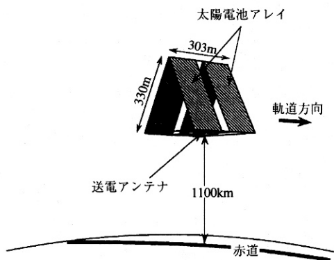
第3図 宇宙科学研究所 太陽発電衛星ワーキンググループが検討を進めている太陽発電衛星SPS2000のモデル。赤道軌道高度1100kmに投入し10MWの電力を地上へ送電する。
