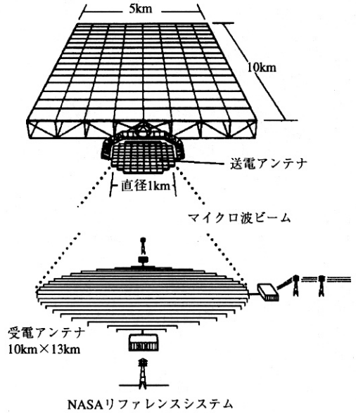
第2図 NASAの太陽発電衛星概念図(リファレンスシステム)。 1基の大きさは5km×10km、出力は5GW。静止衛星軌道に60基配置し、総発電量300GWを想定した。
