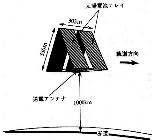
図2. SPS2000システム概念図
