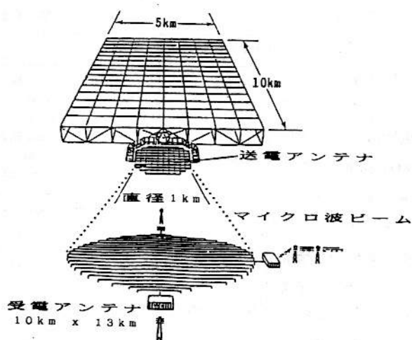
図1. NASAリファレンスシステム
